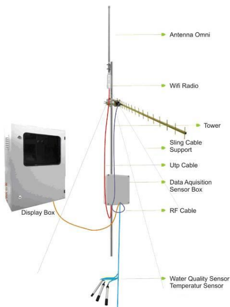
Gambar 5. Stasiun Perantara.
