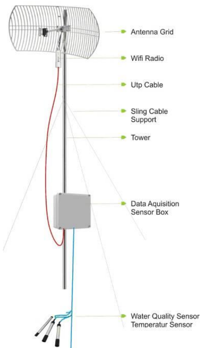
Gambar 3. Stasiun Pengukuran.
